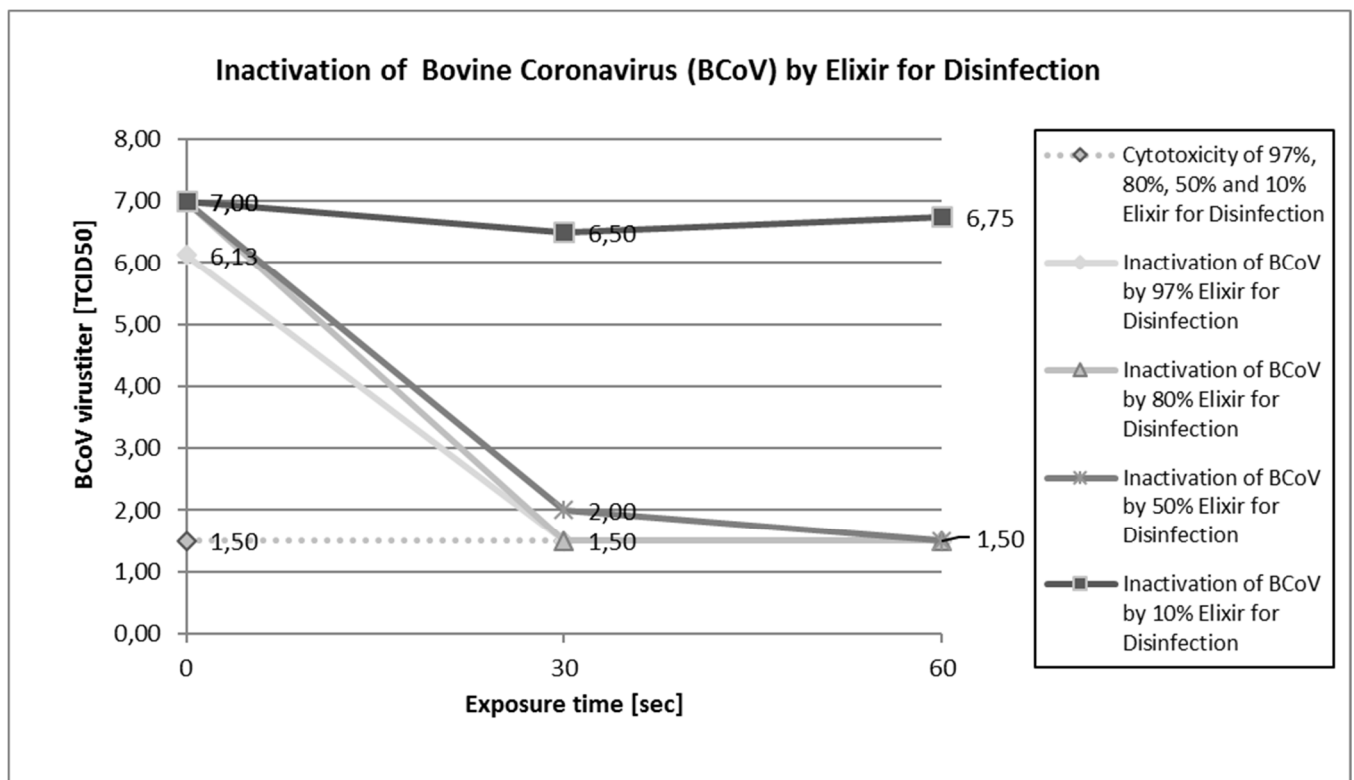
Abb. 2 / fig. 2 : Inaktivierung von Bovinem Coronavirus durch Elixir for Disinfection / inactivation of Bovine Coronavirus by Elixir for Disinfection
